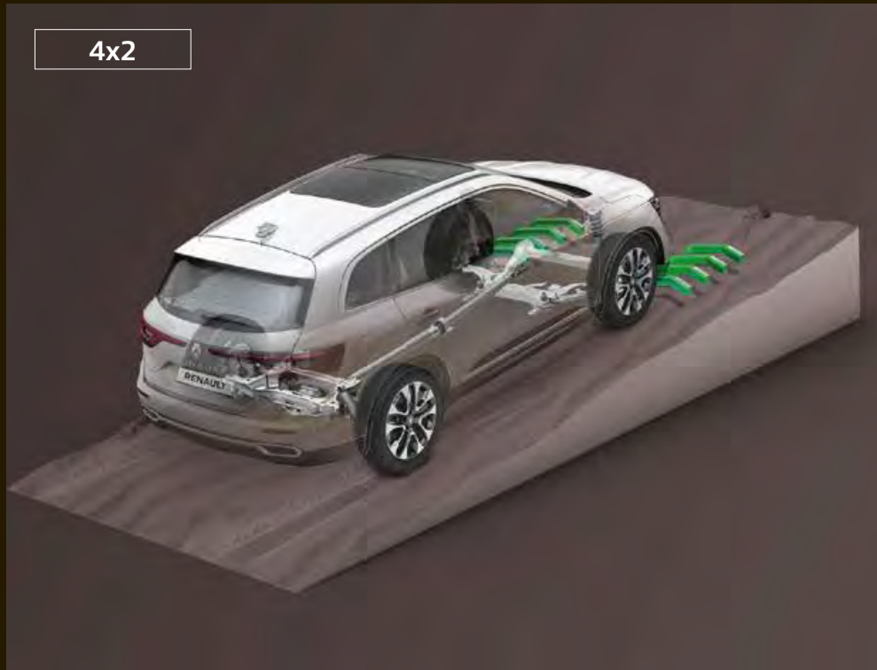
4x2-es hajtásképlet: a hajtás az első kerekeken van
